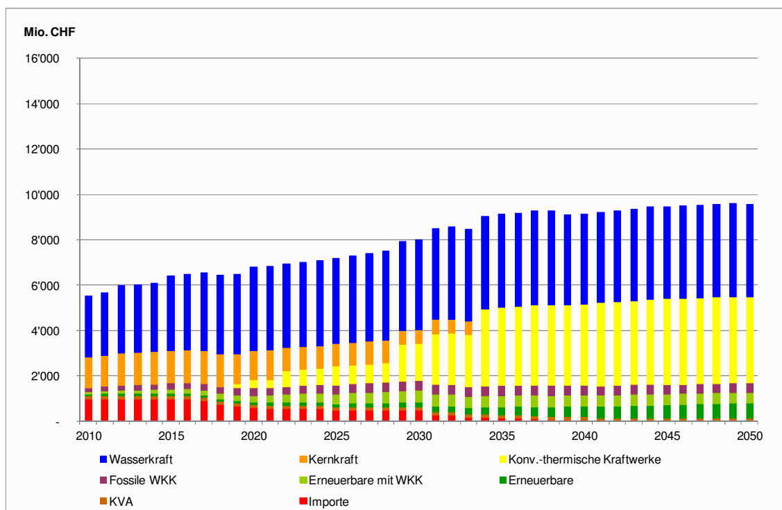
Figur 7-64: Szenario „Weiter wie bisher“, Variante C Jahreskosten des Kraftwerkpark, in Mio. CHF/a
