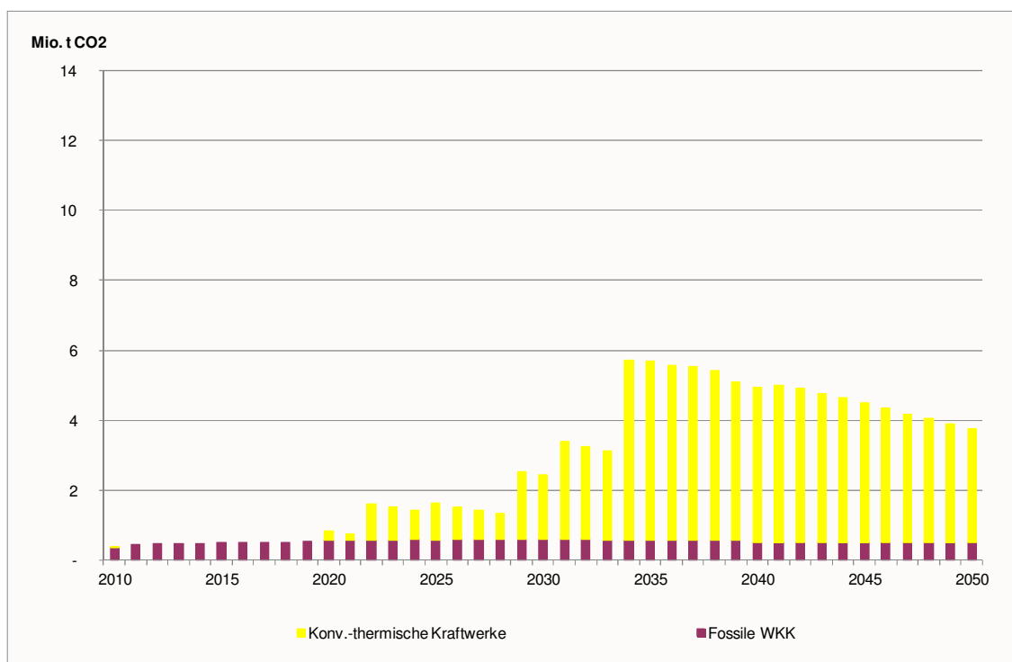
Figur 8-59: Szenario „Neue Energiepolitik“, Variante C CO 2 -Emissionen inkl. Wärmegutschriften, hydrologisches Jahr, in Mio. t CO 2 /a
