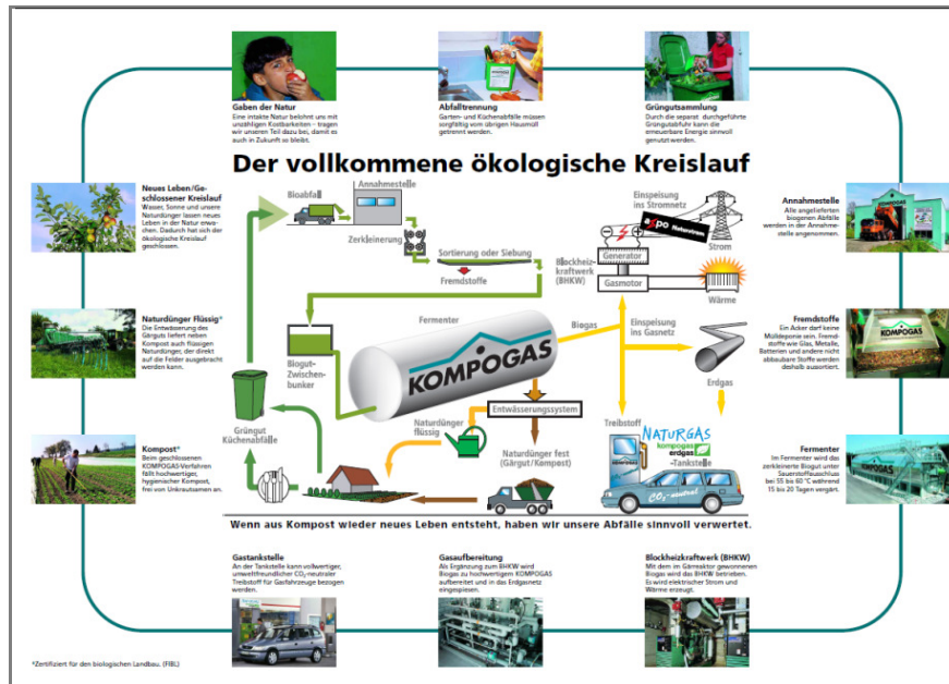
Figur II.1a-5: Verfahrensbild zur Bioabfallvergärung nach dem KOMPOGAS-Verfahren
