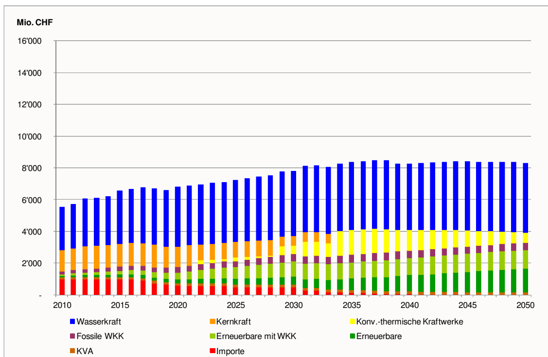
Figur 8-64: Szenario „Neue Energiepolitik“, Variante C&E Jahreskosten des Kraftwerkparcs, in Mio. CHF/a
