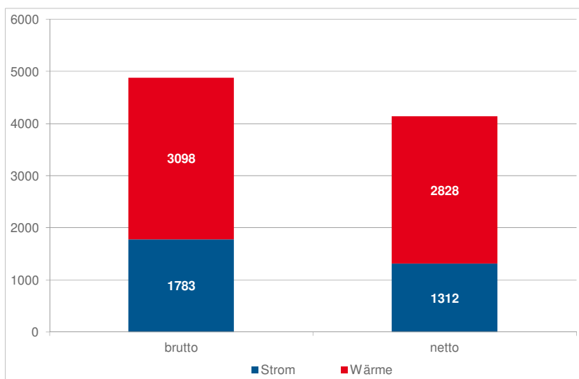
Figur II.1a-4: Energieproduktion aus Schweizer KVA 2009 [GWh]
