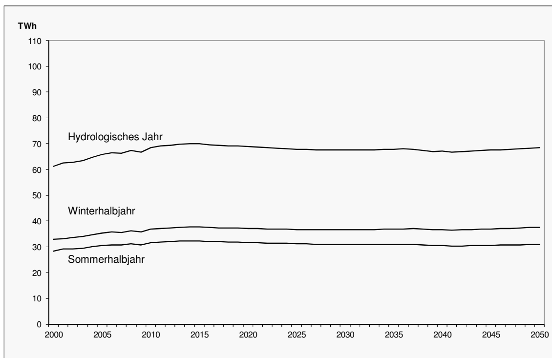
Figur 9-37: Szenario „Politische Massnahmen“ Gesamte Elektrizitätsnachfrage 2000 bis 2050, in TWh_{el}
